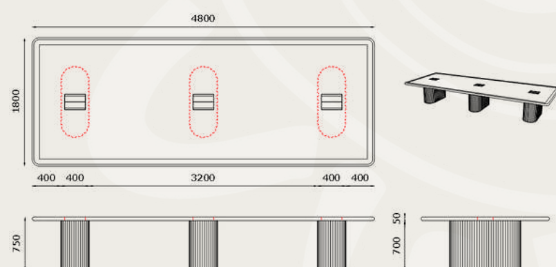
Naarm Table, with Power Box, 4800 x 1200 NAAR-TB-WP-4812
