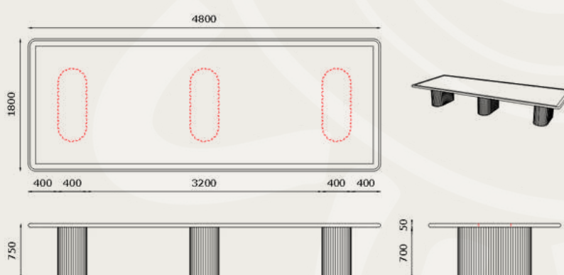
Naarm Table, 4800 x 1800 NAAR-TB-NP-4818
